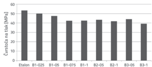
Slika 10. Rezultati ispitivanja čvrstoće na tlak
