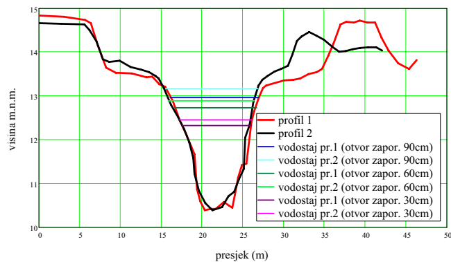
Slika 9. Poprečni presjeci susjednih profila 1 i 2 s izmjerenim vodostajima za razne protoke
