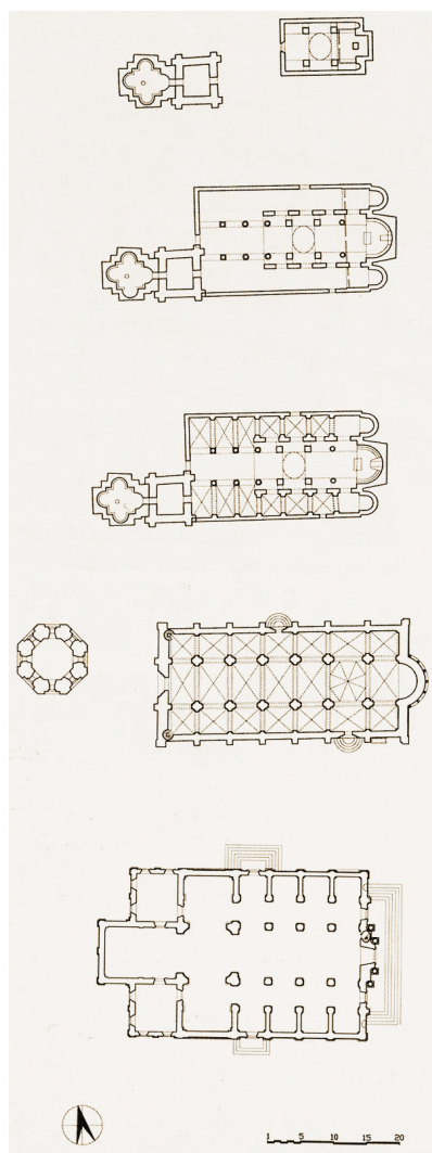
Gradjevni razvoj dubrovačke katedrale (Ž. Peković). Od vrha prema dolje: Sv. Vlaho 972. godine, Sv. Vlaho 1020., Sv. Vlaho 1060., Sv. Marija Velika 12. st., Sv. Marija Velika 17. st.
