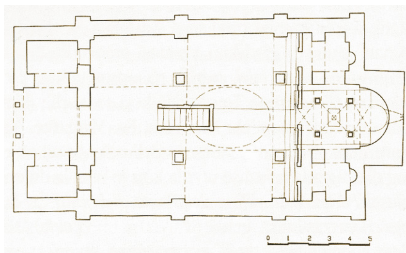
Rekonstrukcija tlocrta crkve Sv. Petra Velikog
