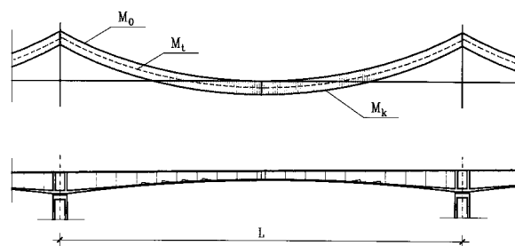
Slika 11. Granična područja momentnog dijagrama pri konzolnoj izvedbi
